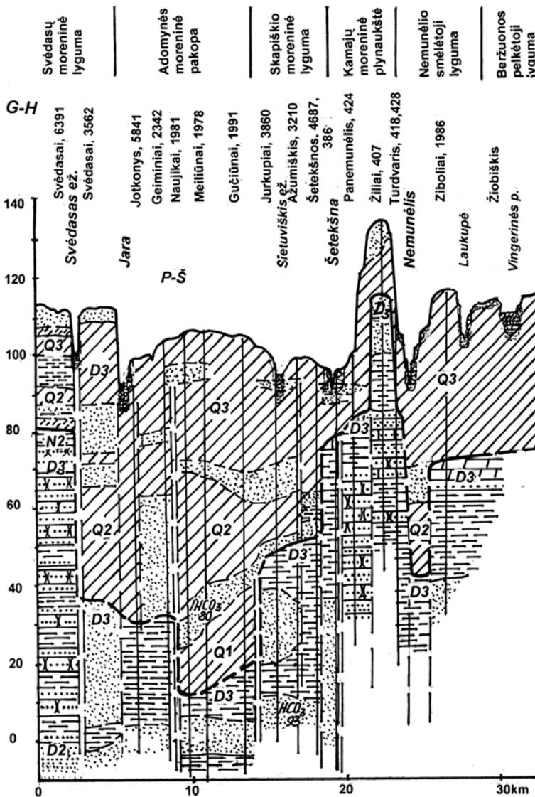
14 pav. Vakarų Aukštaičių plynaukštės vakarinis platuminis geologinis profilis G-H
