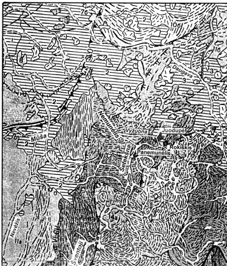
3 pav. Vonsavičius V. (red.) ir Vaitonis V. (papild. žemėlapiu autorius). Tarybinių Pabaltijo respublikų kvartero geologinis žemėlapis. M 1:500 000 (Geological map of the Quaternary deposits of the Soviet Baltic Republic), Leningradas, 1980
