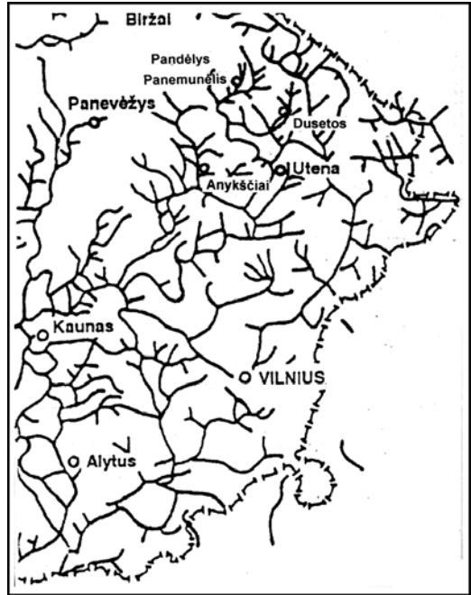
6 pav. Palaidotųjų glacigeninių įrėžių ir senslėnių tinklas rytinėje Lietuvos dalyje pagal A. Šliaupą, 1997, 2000
