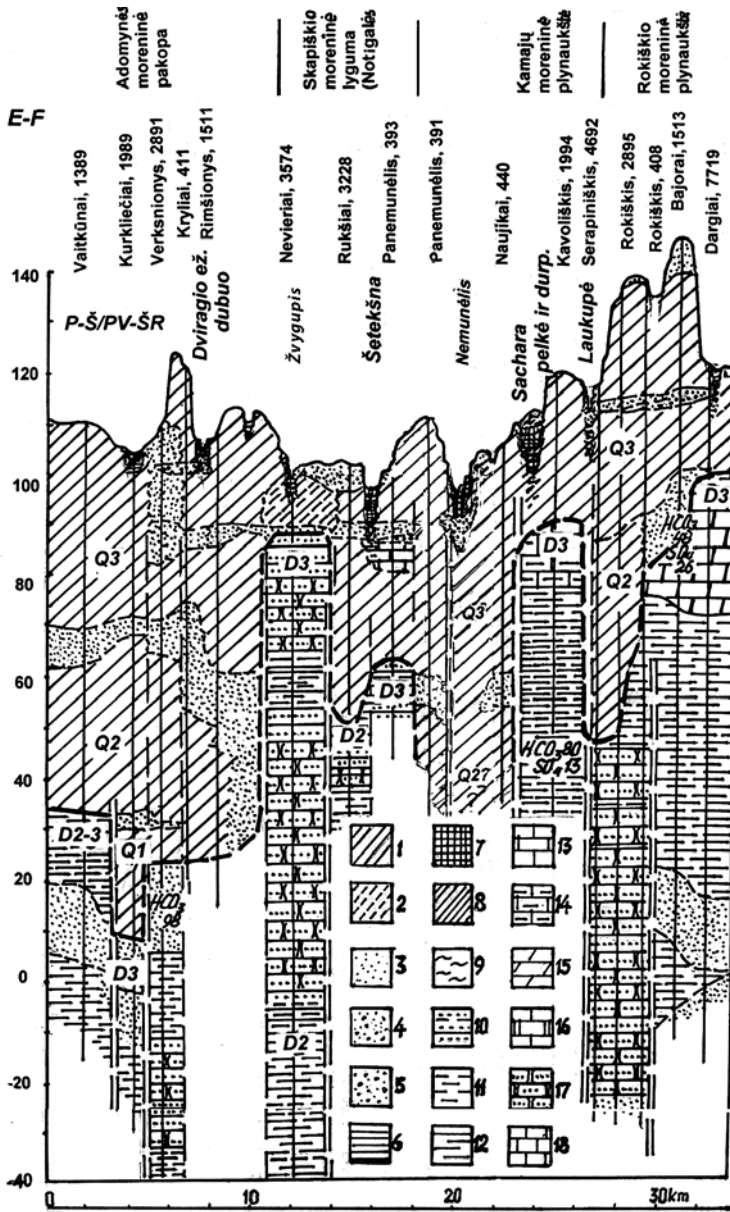
13 pav. Vakarų Aukštaičių plynaukštės rytinis platuminis geologinis profilis E-F Sutartiniai ženklai: 1 – moreninis priemolis su žvyru, smėliu, rieduliais, 2 – moreninis priemolis, 3 – smulkus smėlis, 4 – įvairiagrūdis smėlis, 5 – žvyras su gargždu, 6 – molis, 7 – ežerų sapropelis (molinis, smėlinis, karbonatinis, detritinis), 8 – žemapelkės durpės, 9 – aukštapelkės durpės, 10 – smėlingas molis, 11 – aleuritas, 12 – molis iš pokvarterinių sluoksnių, 13 – klintys, 14 – molingos klintys, 15 – dolomitas, 16 – klintingas dolomitas, 17 – smiltainis, 18 – kreida
