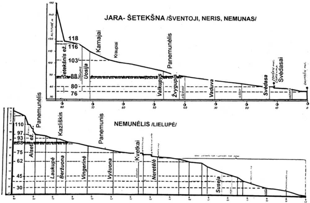
20 pav. Šetekšnos (Jaros) ir Nemunėlio upėkritis, arba išilginiai, profiliai. Stora horizontali punktyrinė linija žymi bendro Nemunėlio–Šetekšnos senslėnio dugno lygį (88 m NN) vėlyvojo ledynmečio pabaigoje
