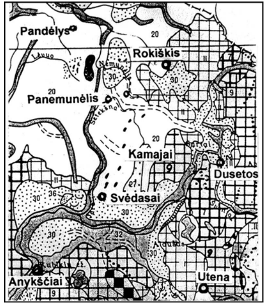
8 pav. Panemunėlio ir gretimų vietovių (Šetekšnos ir Nemunėlio aukštupių baseinų) geomorfologiniai bruožai pagal A. Basalyką, 1962, 1967, 1981
