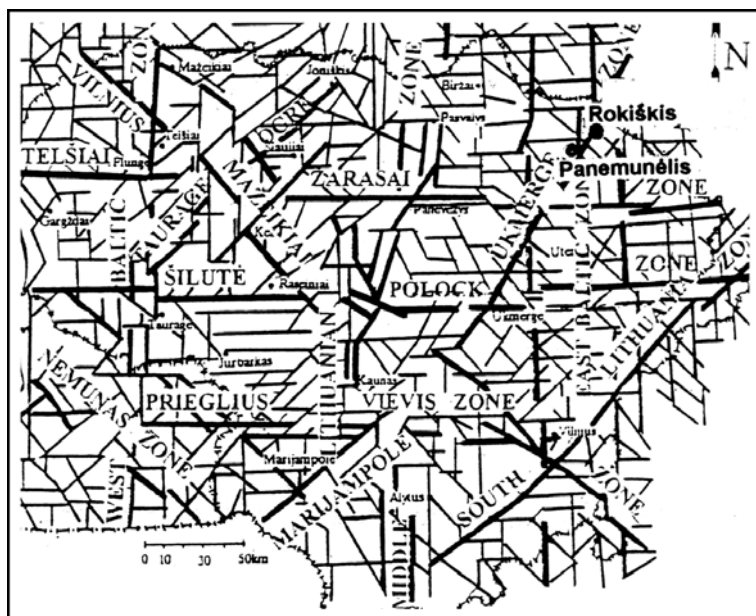
2 pav. Lietuvos neotektoninių aktyviųjų zonų principinė schema. Sistemoje paryškintos ir anglų kalba rašomos pagrindinės tarpregioninės tektoninio aktyvumo bei lūžių zonos, priimtos į europinę apyvertą
