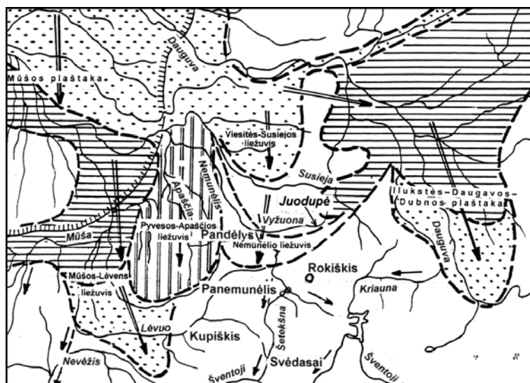
4 pav. Glacimorfologinis žemėlapis, rekonstruojantis nevienalaikius ledyno liežuvius, jų formuotas vietas. Tai V. Vaitonio žemėlapiu, panaudojusio vidutinius ir smulkius lineamentus (giluminių ir paviršiaus struktūrų linijas), koncepcijos pratęsimas ir papildymas Šiaurės Rytų Lietuvos organogeninių klodų duomenimis (Kunskas, 2002)
