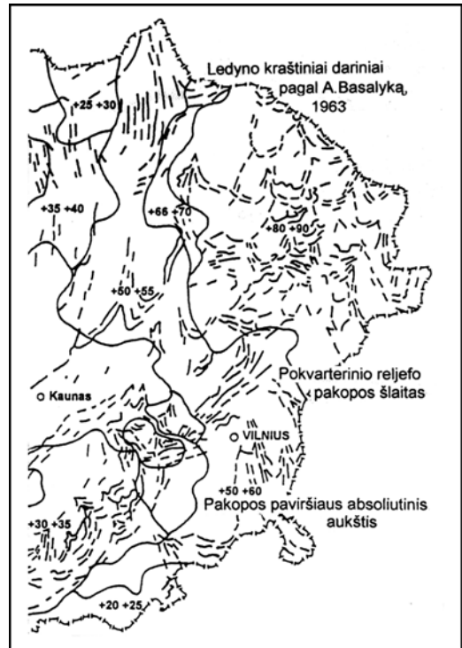
7 pav. Pokvarterinio paviršiaus pakopos ir jų sąryšis su ledyno kraštiniais dariniais (A. Šliaupos ir A. Basalyko koncepcijų sulyginimas (2000))
