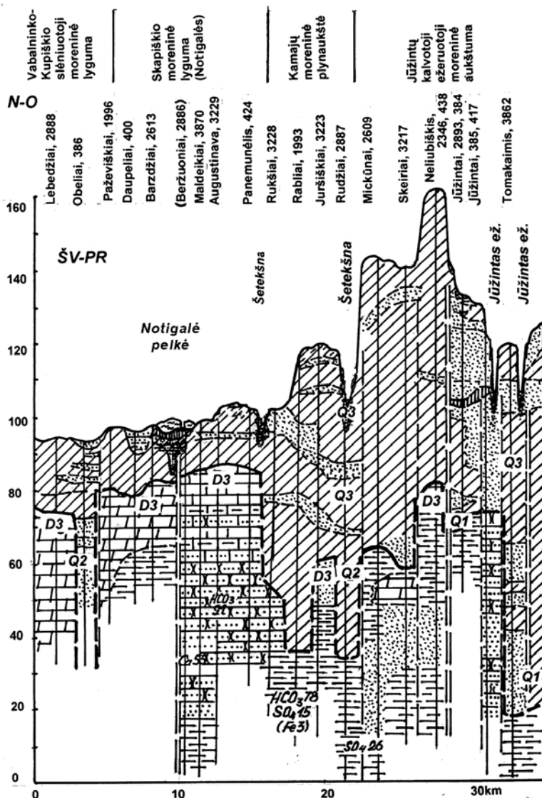
15 pav. Vakarų Aukštaičių plynaukštės geologinis profilis N-O į Aukštaičių aukštumos šlaitą
